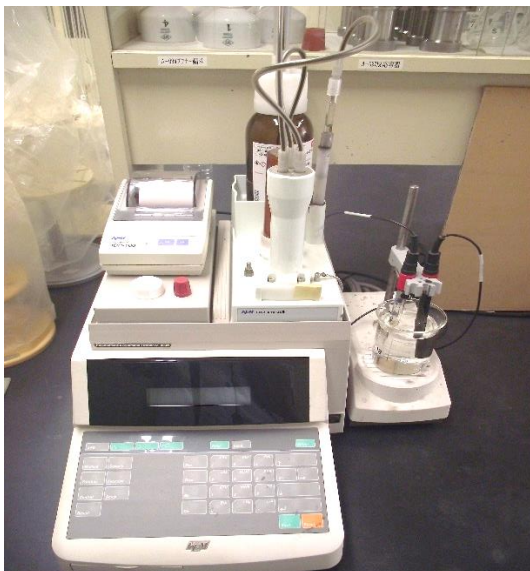
■ 電位差滴定装置
